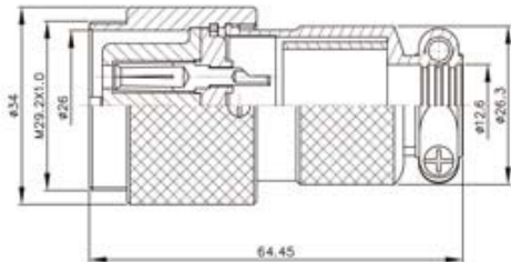
PLT-30-ADF
